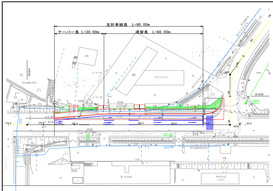
工事計画平面図
